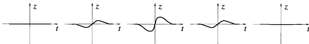
Fig. 7. – The function \zeta .
