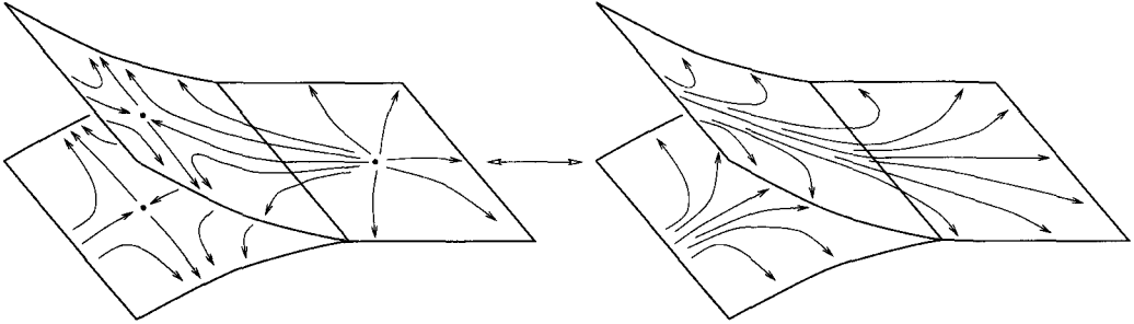
Fig. 5. - Branched elimination lemma I.
